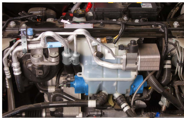
Pompes de refroidissement (bleues) dans la Tesla Model 3
