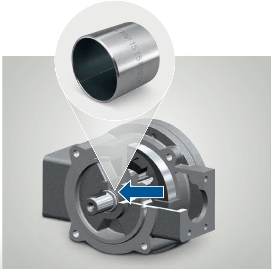
Dişli çarklı pompa kullanımı, PERMAGLIDE® P10 kaymalı yataklar aracılığıyla yataklama (ok)
