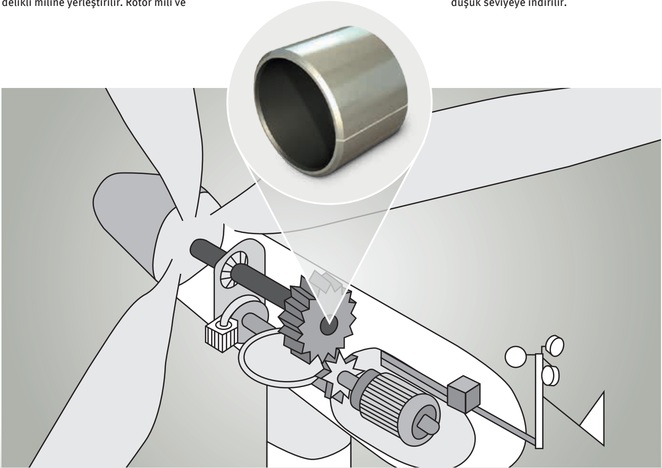
PERMAGLIDE® P10 kaymalı yataklar, rüzgar türbinlerindeki şanzımanların rotor milinde kılavuz yatak olarak kullanılır
