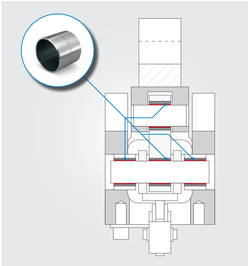
Suspensión del bulón en tensores de palanca articulada con casquillos de cojinete KS PERMAGLIDE®, tipo de construcción PAP ... P10
