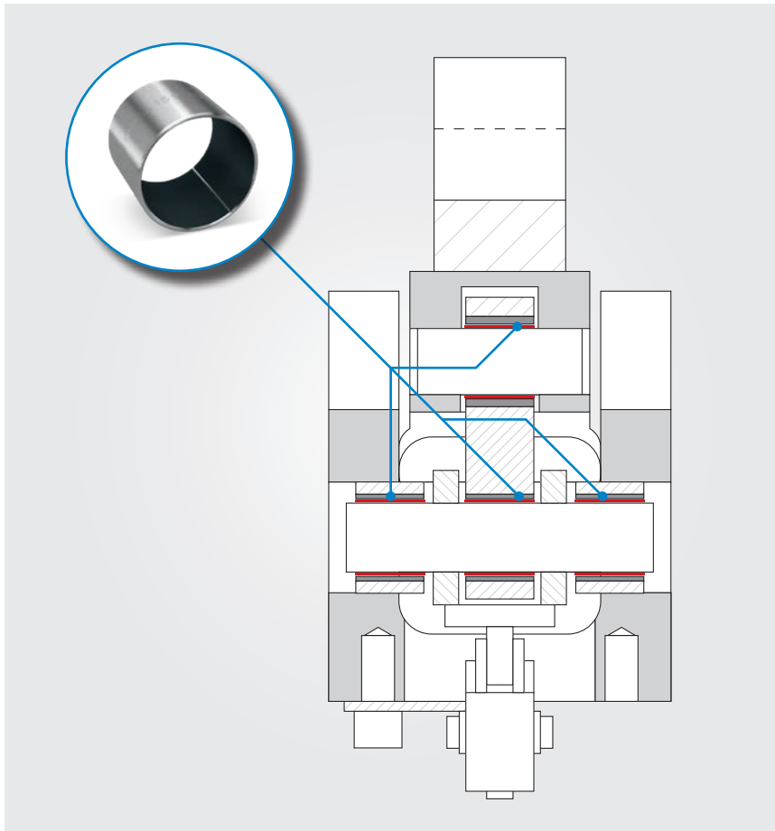
Suspensión del bulón en tensores de palanca articulada con casquillos de cojinete Permaglide®, tipo de construcción PAP ... P180
