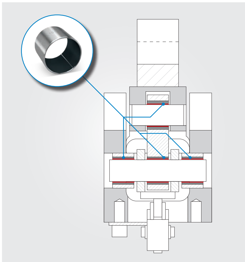
Palier d'axe dans des systèmes à genouillère avec des bagues de coussinet Permaglide® du type de construction PAP ... P180
