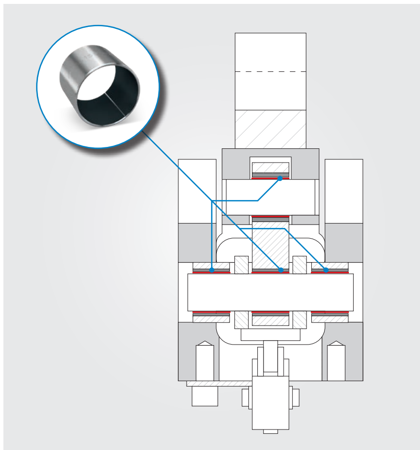
łożyskowanie sworzni w zaciskach kolanowych tulejami łożysk ślizgowych Permaglide® typu PAP ... P180
