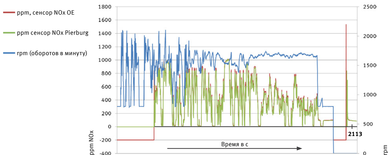
Рис. 1: Сравнение производительности сенсоров NOx Pierburg и сенсоров OE
