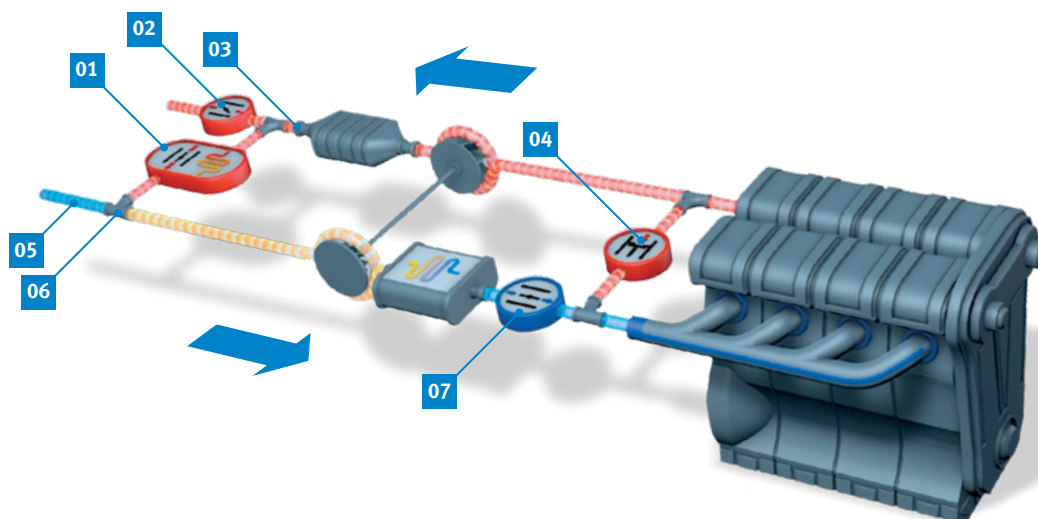
01 VÁLVULAS EGR (BP)
