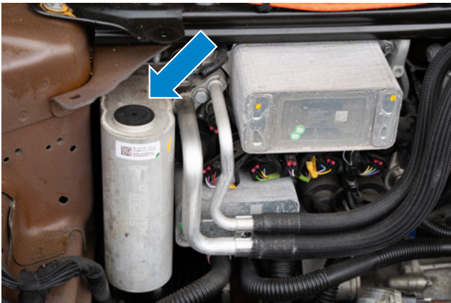
Posición de montaje en el supercolector del Model 3
