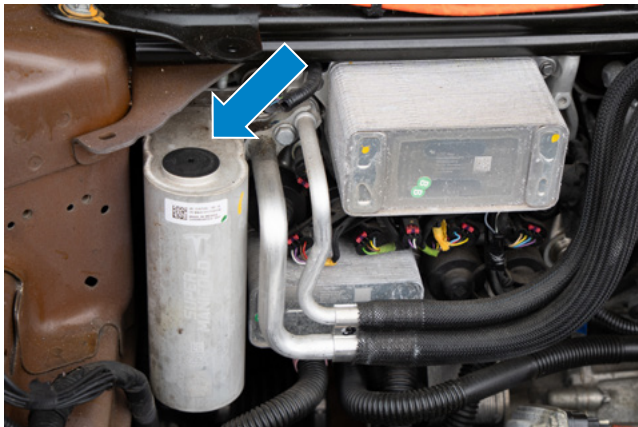
Situation de montage dans le Supermanifold du Model 3
