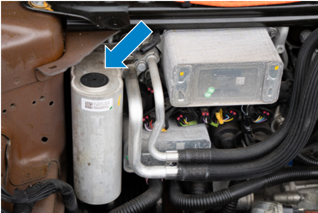
Sytuacja montażowa w supermanifold w Modelu 3
