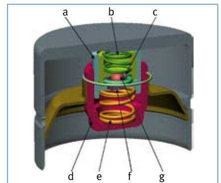
Abb.3 Bestandteile Leerhubtassenstößel: a) Innere Kolben e) Rückstellfeder b) Feder f) Feder c) Ventilkappe g) Kugel d) Äußerer Kolben [Bild: INA]
