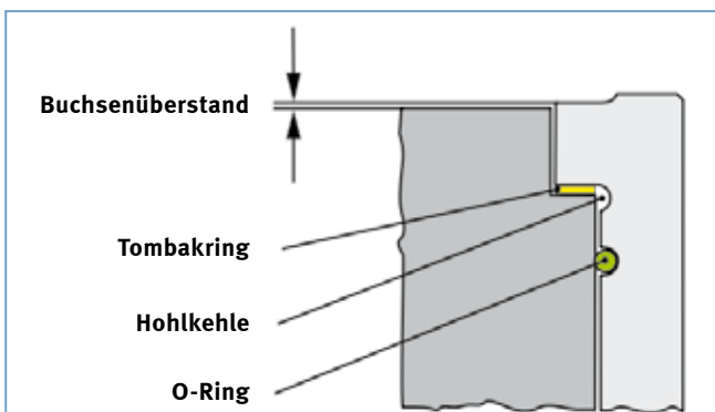
Abb. 1 Zylinderbuchsen-Abdichtung [© MS Motor Service International GmbH]
