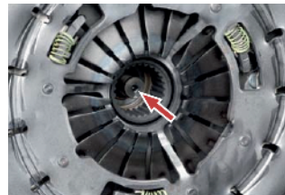
Foto 2: 415 0377 10 z zamocowanym sprzęgłem (SAC)
