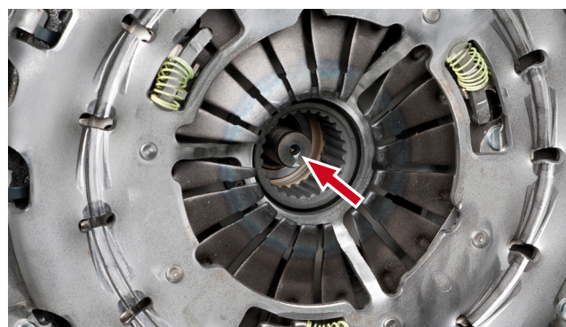
Рисунок 2: 415 0377 10 с установленным сцеплением (SAC)
