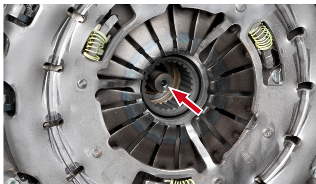
Bild 2: 415 0377 10 med monterad koppling (SAC)
