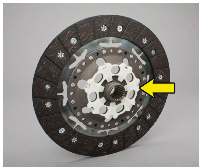
Obrázek 1: LuK spojková lamela s plastovým kroužkem
