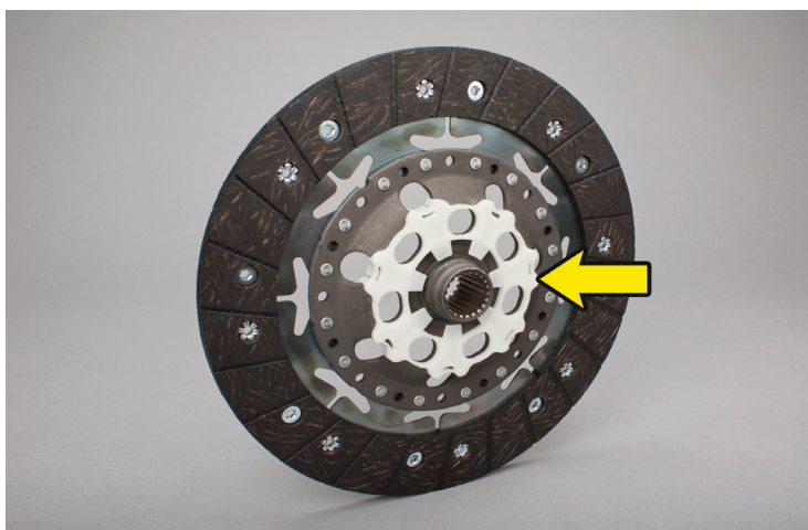
איור 1: דיסק מצמד בעל טבעת פלסטיק
