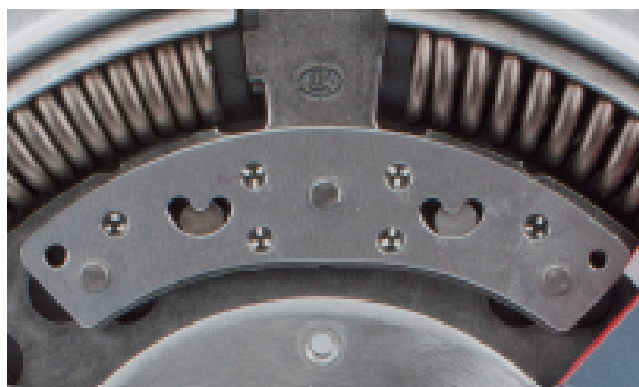
Foto2: Element wahadła
