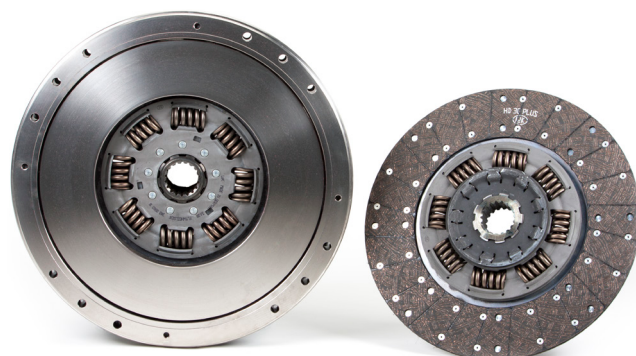
Снимка 2: LuK двойно дисков съединител с един и същ профил на главините
