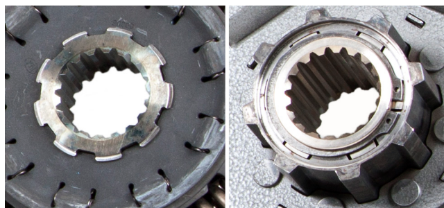
Снимка 1: LuK главина (вляво), главина на друг доставчик (вдясно)
