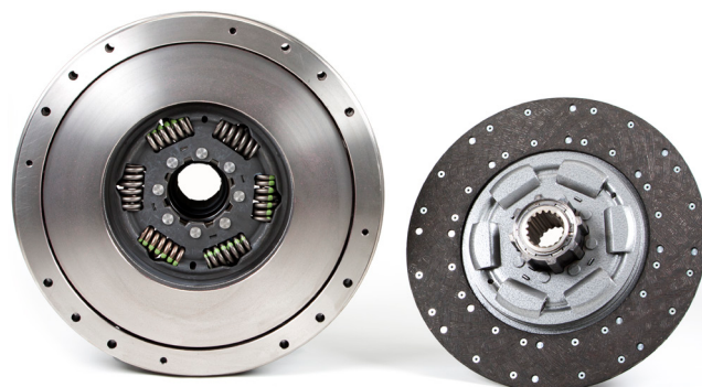
Снимка 3: Пример за двойно дисков съединител с различен дизайн на главините
