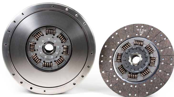
איור 2: מצמד בעל דיסק כפול מתוצרת LuK בעל אותו פרופיל טבור
