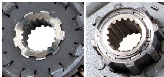
איור 1: טבור מתוצרת LuK (שמאל), טבור מתוצרת חברה אחרת (ימין)
