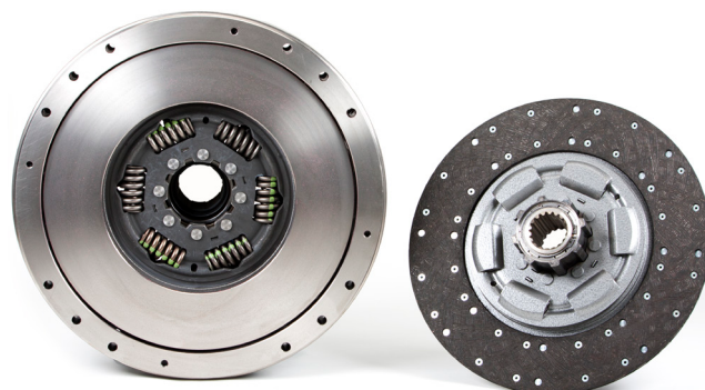
3. ábra: Példa egy eltérő agykialakítású kéttárcsás kuplungra
