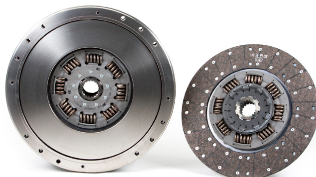
2. ábra: LuK kéttárcsás kuplung azonos agyprofillal
