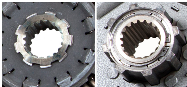
1. ábra: LuK-agy (bal), más gyártó agya (jobb)
