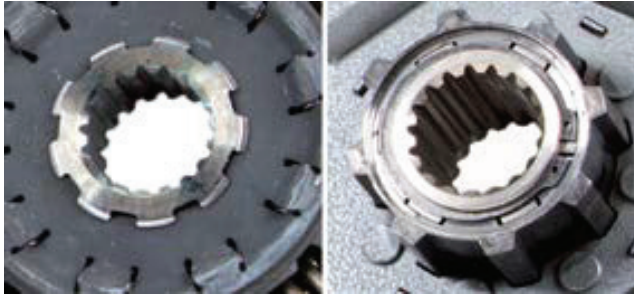
Resim 1: LuK debriyaj göbeği (sol), başka bir tedarikçinin debriyaj göbeği (sağ)
