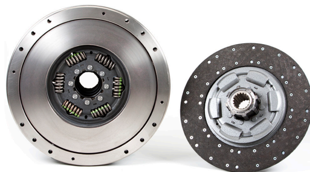
Зображення 3: Приклад двудискового зчеплення з неоднаковою конструкцією ступиць дисків зчеплення
