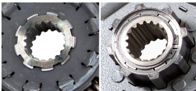
Зображення 1: Ступиця LuK (зліва), ступиця іншого виробника (справа)
