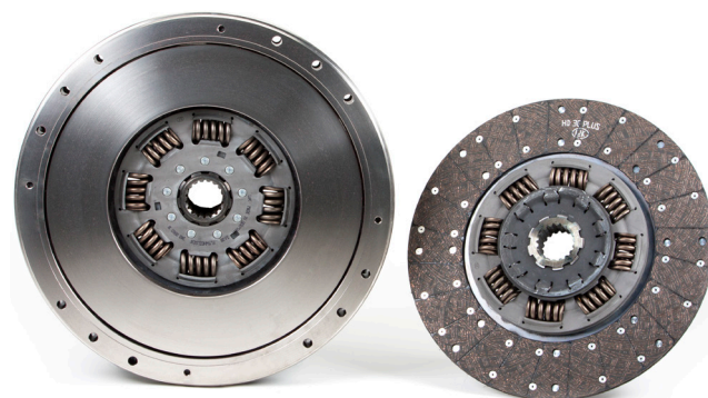
Зображення 2: Двудискове зчеплення LuK з однаковим профілем шліцьових ступиць
