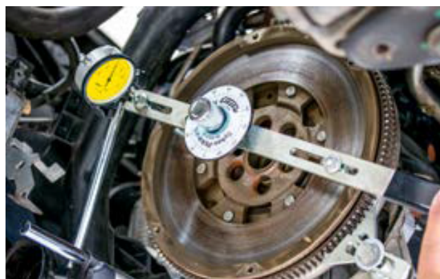
Narzędzie specjalne LuK, nr ref. 400 0080 10
