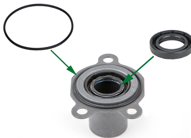
Vodicí pouzdro s předmontovaným O-kroužkem a těsněním hřídele
