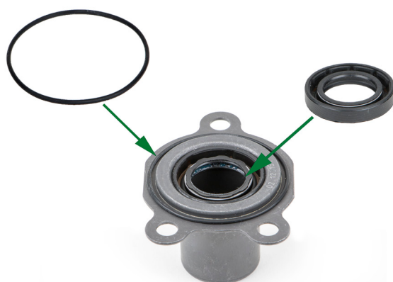
שרוול מוביל בעל טבעת או (אורינג) ואטם ציר המותקנים מראש במפעל הייצור
