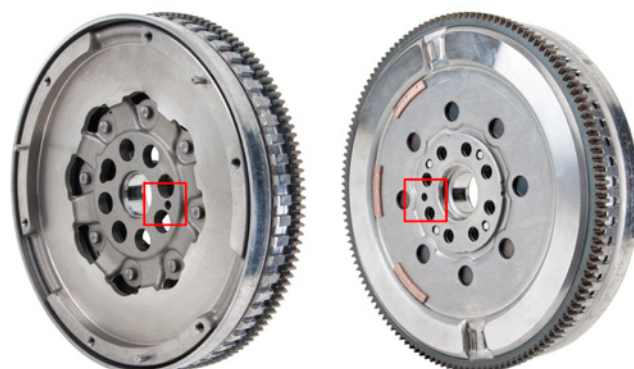
Imagen 1: Marca de referencia en el volante bimasas
