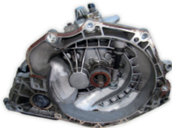
Foto 1: Podczas naprawy sprzęgła należy sprawdzić ułożyskowanie dźwigni, widełek zwalniających
