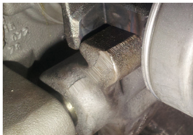
Imagen 2: Horquilla de desembrague con perfil de leva redondeado
