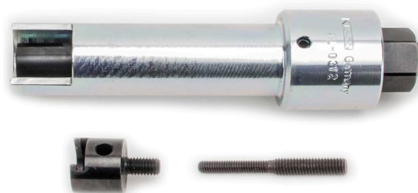
Obrázek 1: Speciální přípravek Klann KL-1600-1610 umožňuje bezproblémovou demontáž
