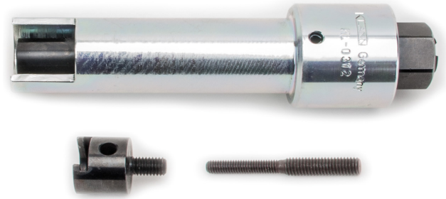
Kuva 1: Erikoistyökalu Klann KL-1600-1610 mahdollistaa ongelmattoman irrotuksen
