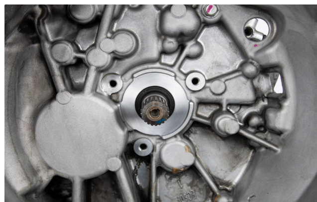
Bild 1: Slavcylinderns kontaktyta i växellådshuset
