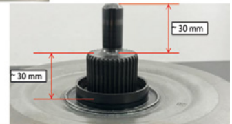
Imagen 3: Dimensiones modificadas en el engranaje y en el pasador guía
