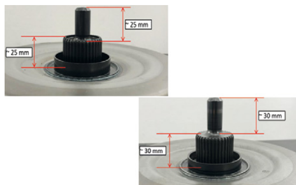
Figure 3 : Modification des dimensions de l'arbre d'entrée et de la douille de guidage
