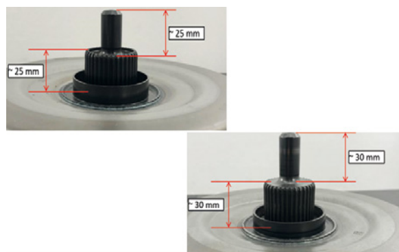
Figura 3: Dimensões modificadas do estriado e do pino guia
