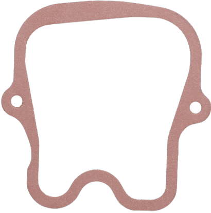
Eski 638.901 – MAN 51.03905.0134 Malzeme: EWP kırmızı (yumuşak malzeme)
