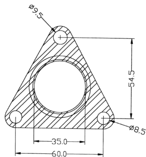
Cotas de la junta
