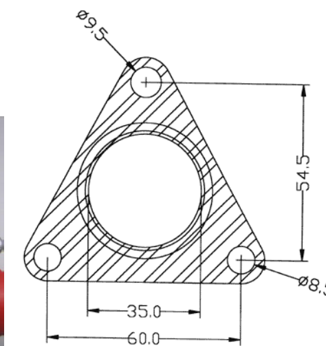
Wymiary uszczelki
