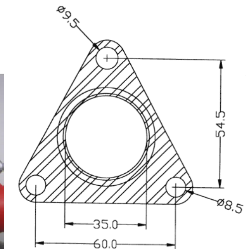
Maße der Dichtung
