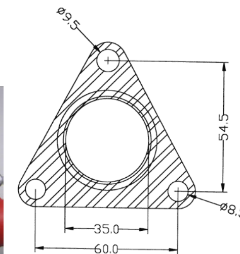
Dimenzije tesnila
