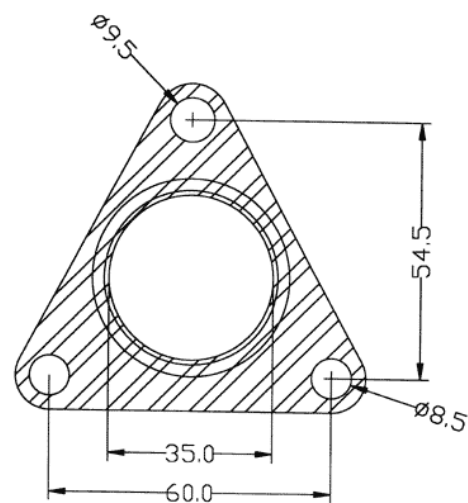
Pakningens dimensioner
