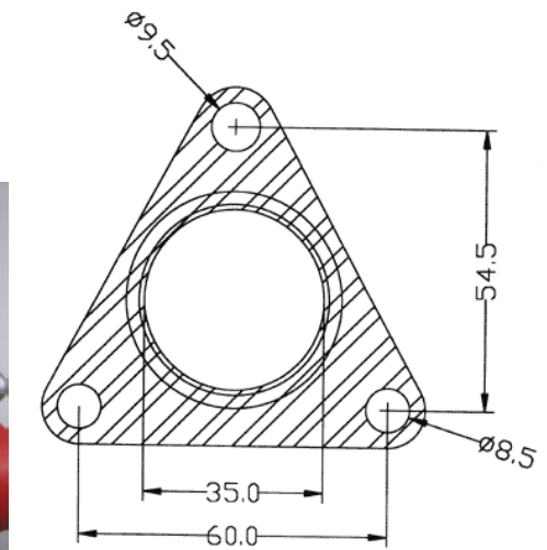
Quote della guarnizione
