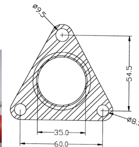
Dimensiunile garniturii de etanșare
