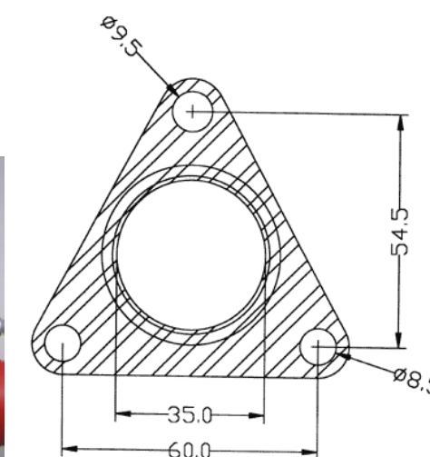
Dimensions du joint
