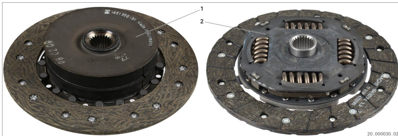
Fig. 1: Clutchskiver Porsche
