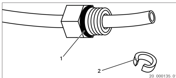
Ábra 9 Szorítódarab eltávolítása
