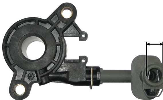
Sl. 2: CSC 3182 600 129 → 3182 654 146 → 3182 654 299 prečnik hidrauličkog priključka 13,3 mm
