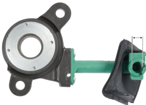
Sl. 3: CSC 3182 600 120 prečnik hidrauličkog priključka 12,2 mm
