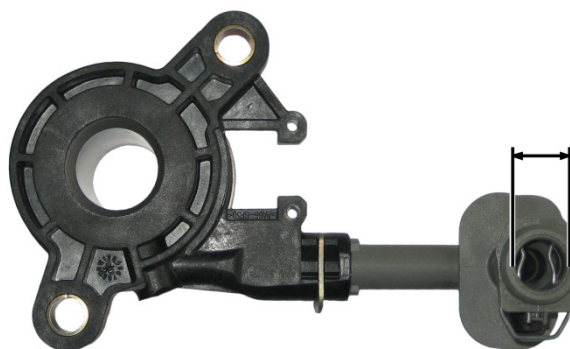
Sl. 2: CSC 3182 600 129 → 3182 654 146 → 3182 654 299 Premer hidravličnega priključka 13,3 mm
