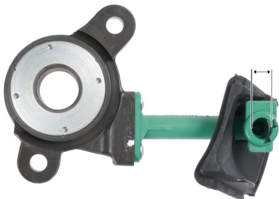
Sl. 3: CSC 3182 600 120 Premer hidravličnega priključka 12,2 mm
