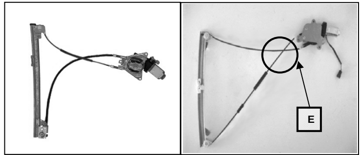
Elevalunas original – lève-vitre original Nuestro elevalunas – notre lève-vitre – oem window regulator – levandator – our window regulator – nosso de vidro original levantador de vidro
