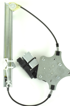
Nuestro Elevallunas / Our window regulator / Notre lève-vitre / Nosso elevador de vidro
