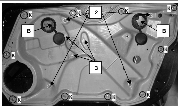
Puerta lado derecho, Portière avant droite, Right front door, Porta frente dirieta
