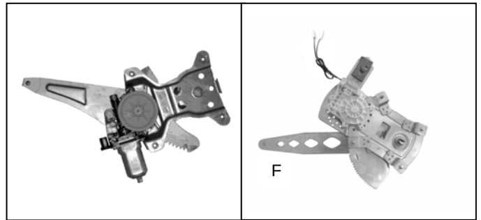
Elevalunas original – lève-vitre original Nuestro elevavinas – notre lève-vitre – oem window regulator – levandator – our window regulator – nosso de vidro original levantador de vidro
