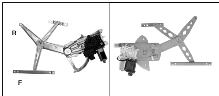
elevavinas original – lève-vitre original Nuestro elevavinas – notre lève-vitre – oem window regulator – levandator – our window regulator – nosso de vidro original levantador de vidro
