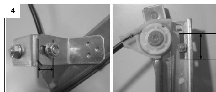
Puerta lado derecho, Portière arrière droite, Right rear door, Porta traseira direita
