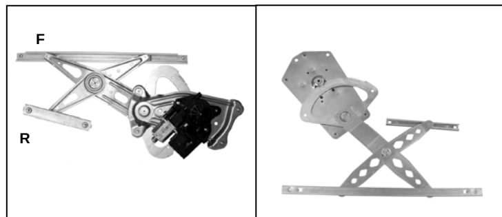
Elevallas original – lève-vitre original Nuestro elevallas – notre lève-vitre – oem window regulator – levandator – our window regulator – nosso de vidro original levantador de vidro
